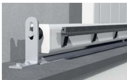
Rail inox + Butée + Roulette pour portail coulissant composée de : • chape alu (couleur portail) • galet inox + Crémaillère en nylon armé pour motorisation
